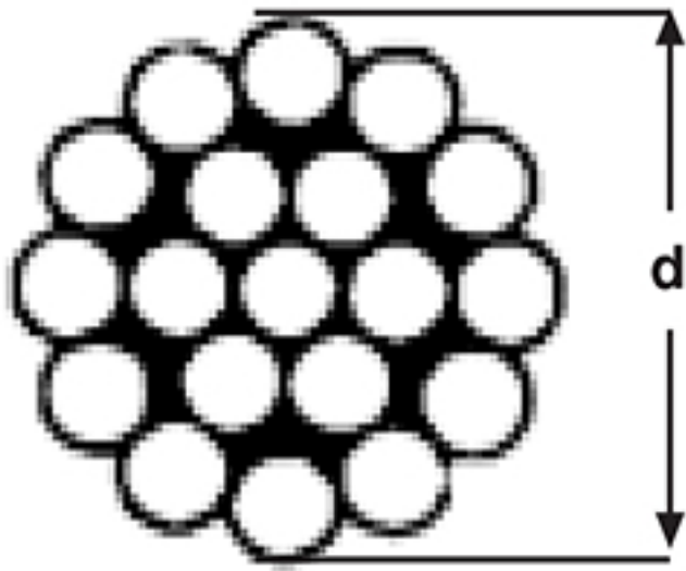
1 x 19 PASLANMAZ ÇELİK HALAT
