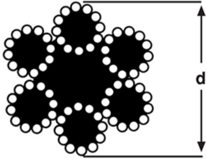
6 X 12 + 7 STANDARD LİF ÖZ
