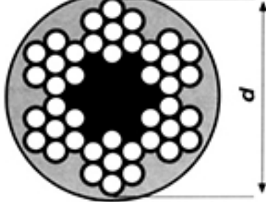
PVC KAPLI ÇELİK HALAT
