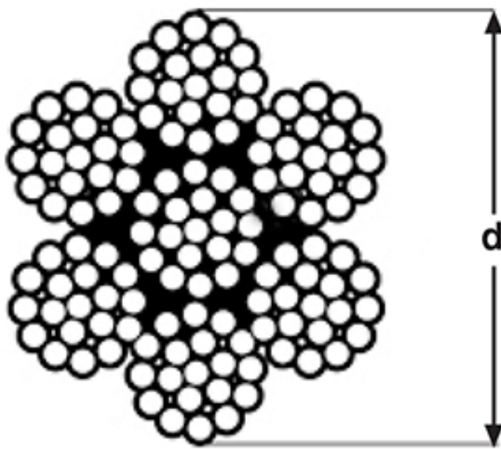
7 X 19 PASLANMAZ ÇELİK HALAT
