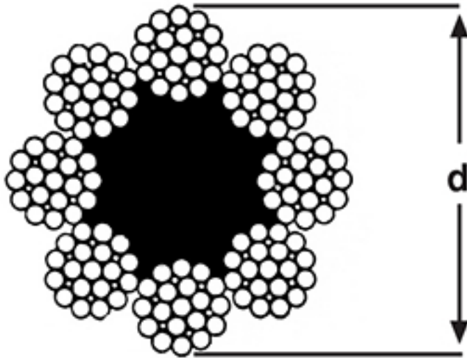
8 X 19 FILLER 8 ( 1 + 6 + 6dt + 12 )
